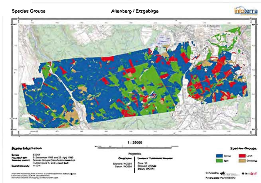
Ejemplo de Aplicación Forestal: mapeo de los grupos de especie arbórea. Área: Altenburg/Erzgebirge, Alemania
