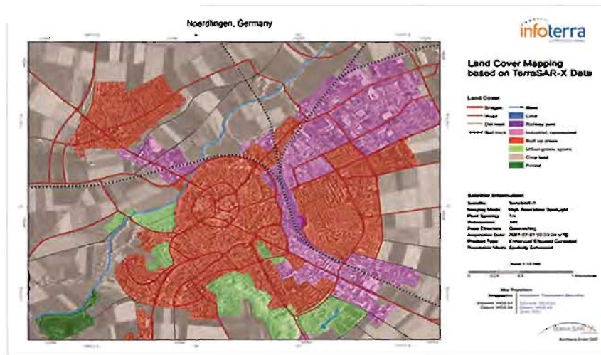
Mapa de alta resolución de cobertura del terreno en Noerdlingen: extracción de información superficial, por ejemplo, para planificación ambiental o espacial. Basado en adquisición TerraSAR-X en modo SpotLight (resolución de 1,3m) Producto preliminar adquirido durante fase de calibración
