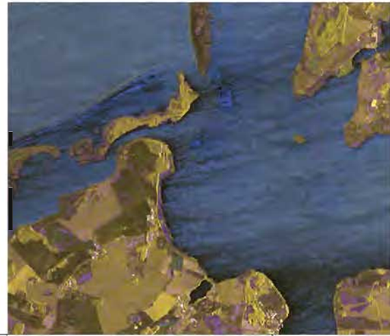
Parte de imagen TerraSAR-X en modo StripMap (Resolución de 3m) de la zona costera Alemana (mar Báltico), imagen en polarización doble, lo que permite por ejemplo, la identificación de tipos de cosecha para aplicaciones agrarias. Producto preliminar adquirido durante fase de calibración
