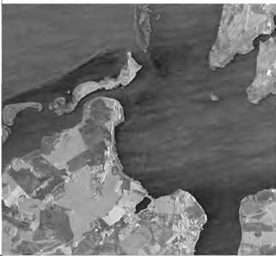
Parte de imagen TerraSAR-X en modo StripMap (Resolución de 3m) de la zona costera Alemana (mar Báltico), imagen en polarización simple. Producto preliminar adquirido durante fase de calibración
